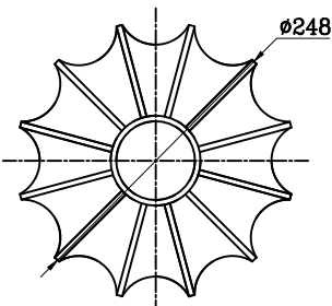
Impeller
