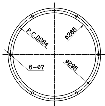
Flange
